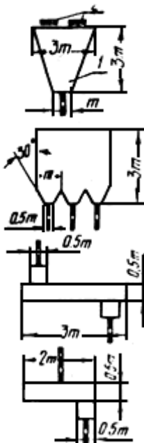
Бункеры пылевидного топлива (длина бункера определяется числом пылепитателей)
